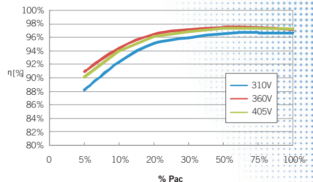
Rendementscurve voor Omniksol 2.0k-TL
